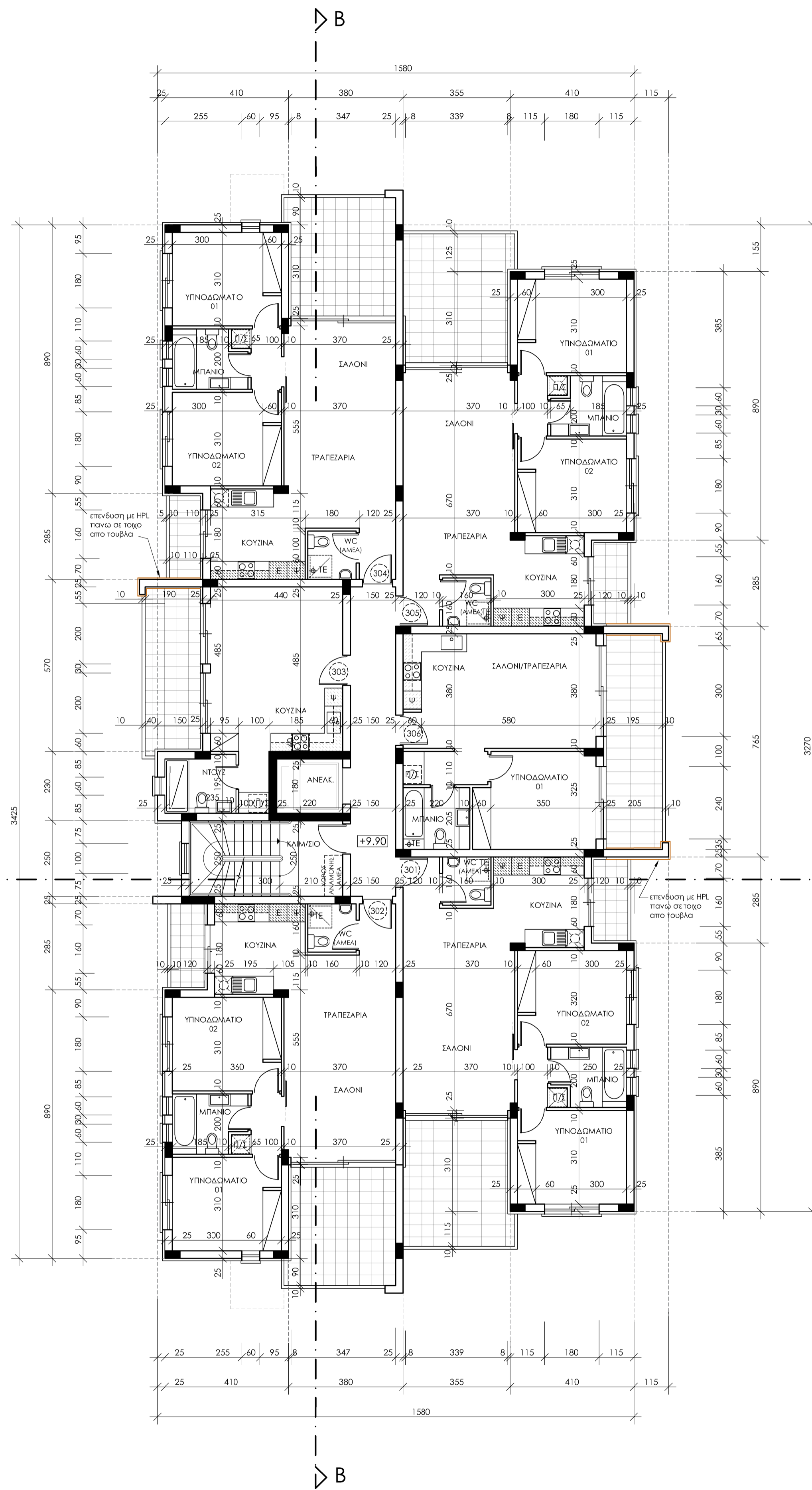
ΚΑΤΟΨΗ 3ου ΟΡΟΦΟΥ BLOCK B
