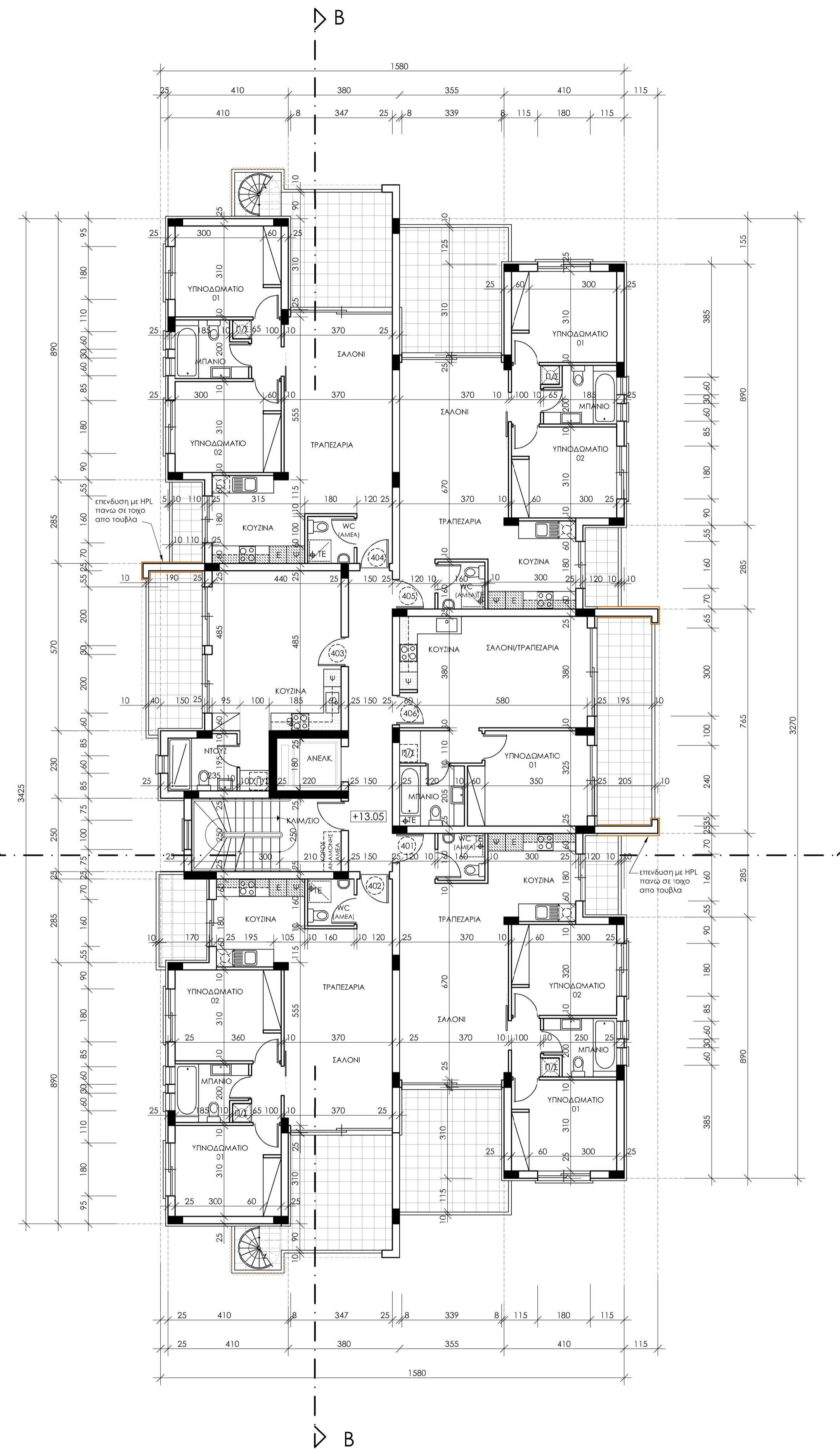
ΚΑΤΟΨΗ 4ου ΟΡΟΦΟΥ BLOCK B
